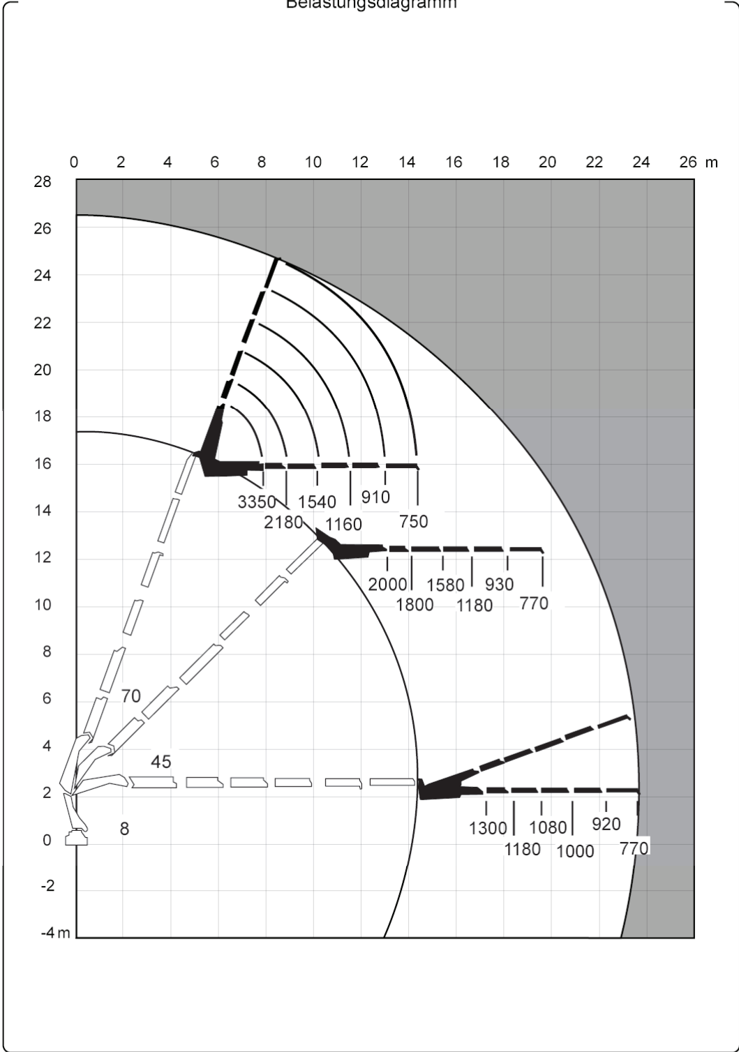
Belastungsdiagramm
